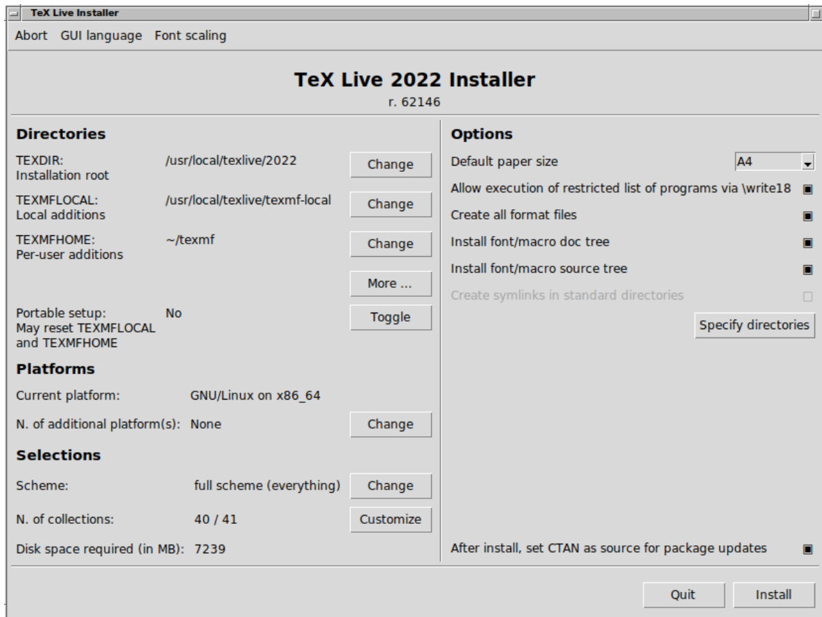
FIGURE 4 – Fenêtre de installateur en mode GUI avancé (GNU/Linux)
